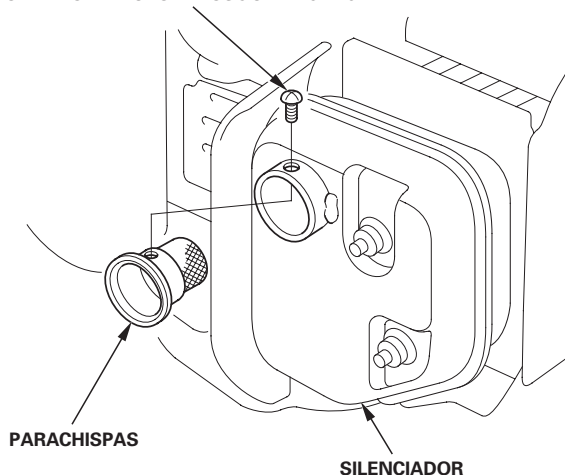
SILENCIADOR
