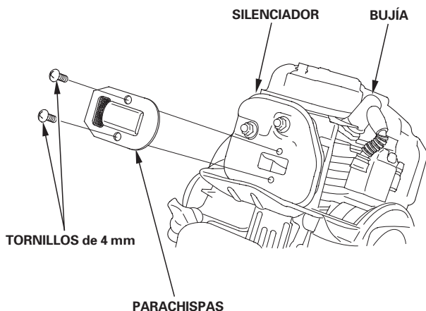
PARACHISPAS
