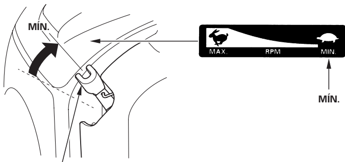
PALANCA DEL ACELERADOR
